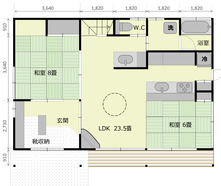
1 F 平面図
